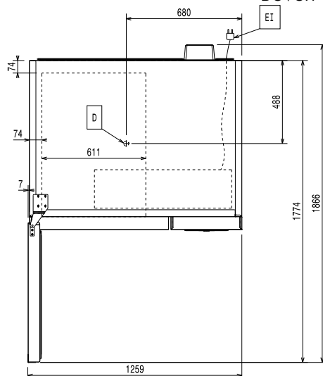
Boven aanzicht
